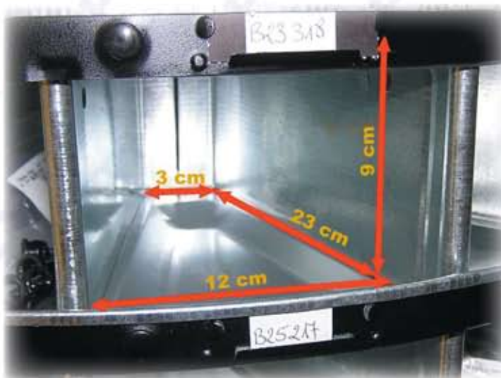
wymiary jednej przegródki
